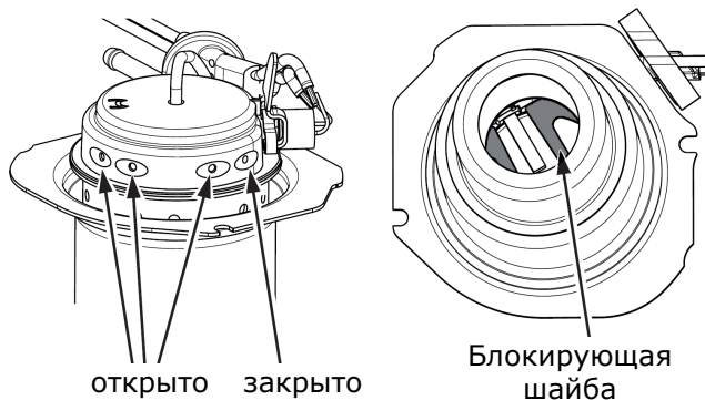
Рис. 904 Бензиновая горелка
