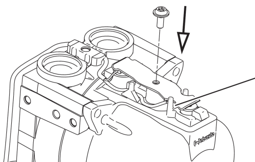
Рис. 920 Установите винты
