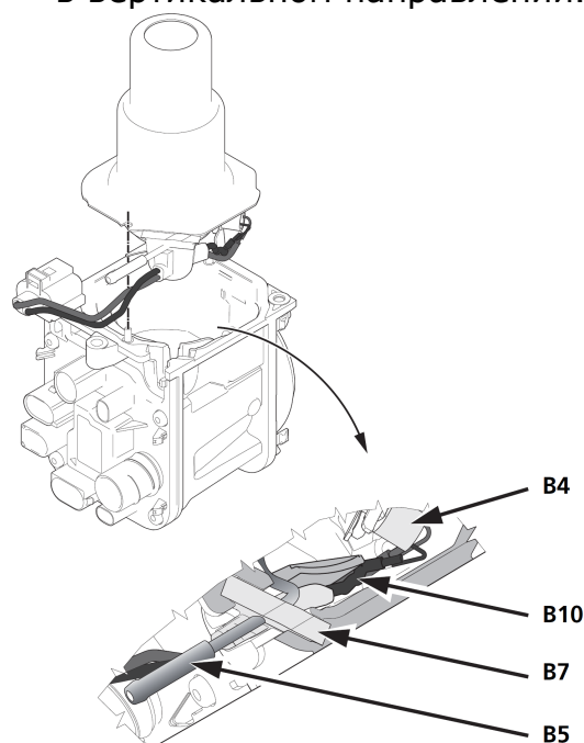
Рис. 903 Детальное представление расположения проводки штифта накала
