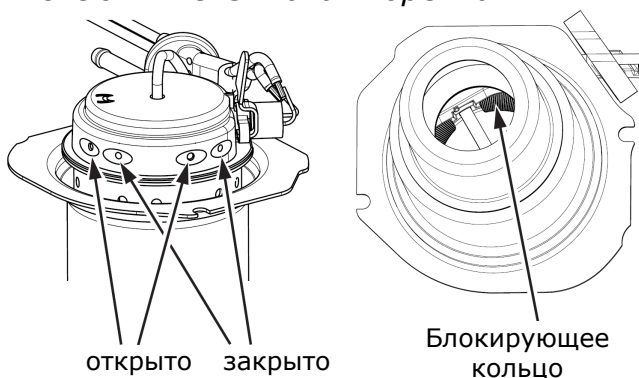
Рис. 905 Дизельная горелка
