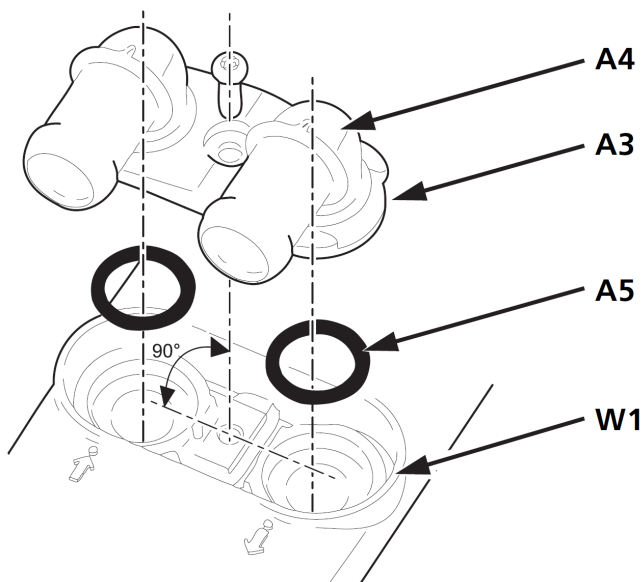
Рис. 924 Установка пластины крепёжной жидкостных патрубков
